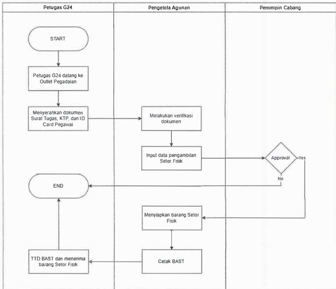
Gambar 2 Alur Proses Serah Terima Setor Fisik Tabungan Emas
